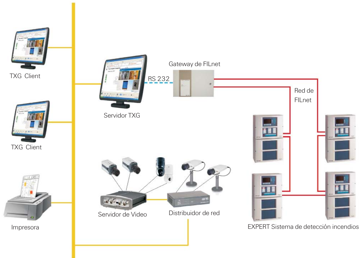
Conectando una red de paneles ZX vía ZX FILNet
